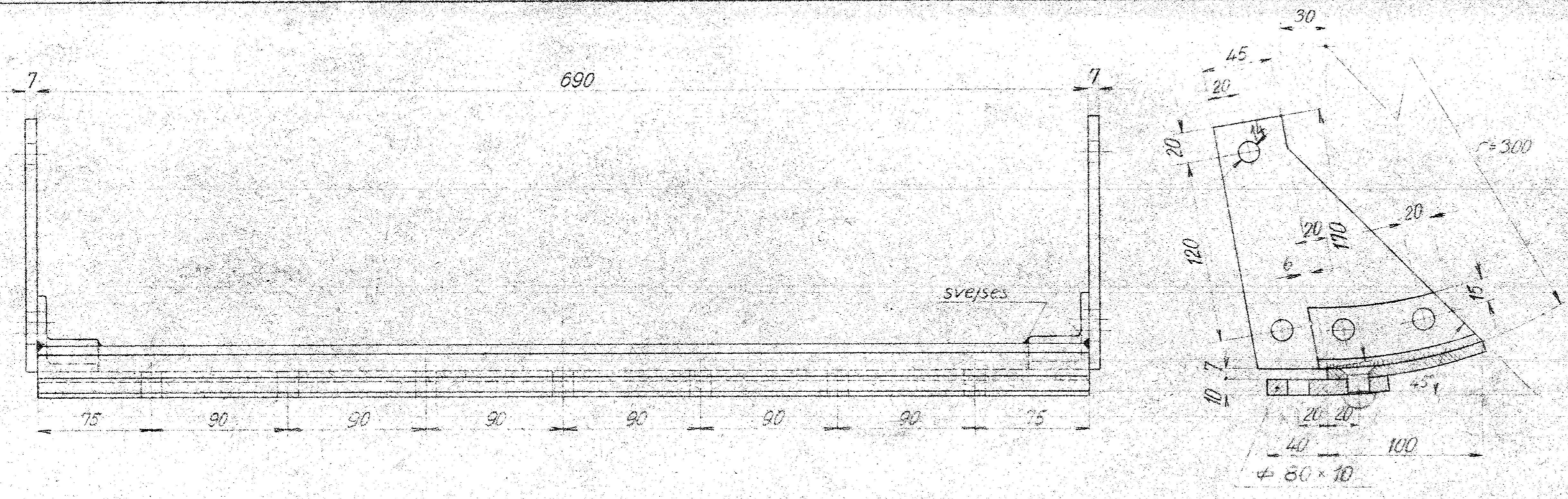
PR 7b Pos 2. Askefang. 1Stk. 1:25 Rev. Flusjern.
