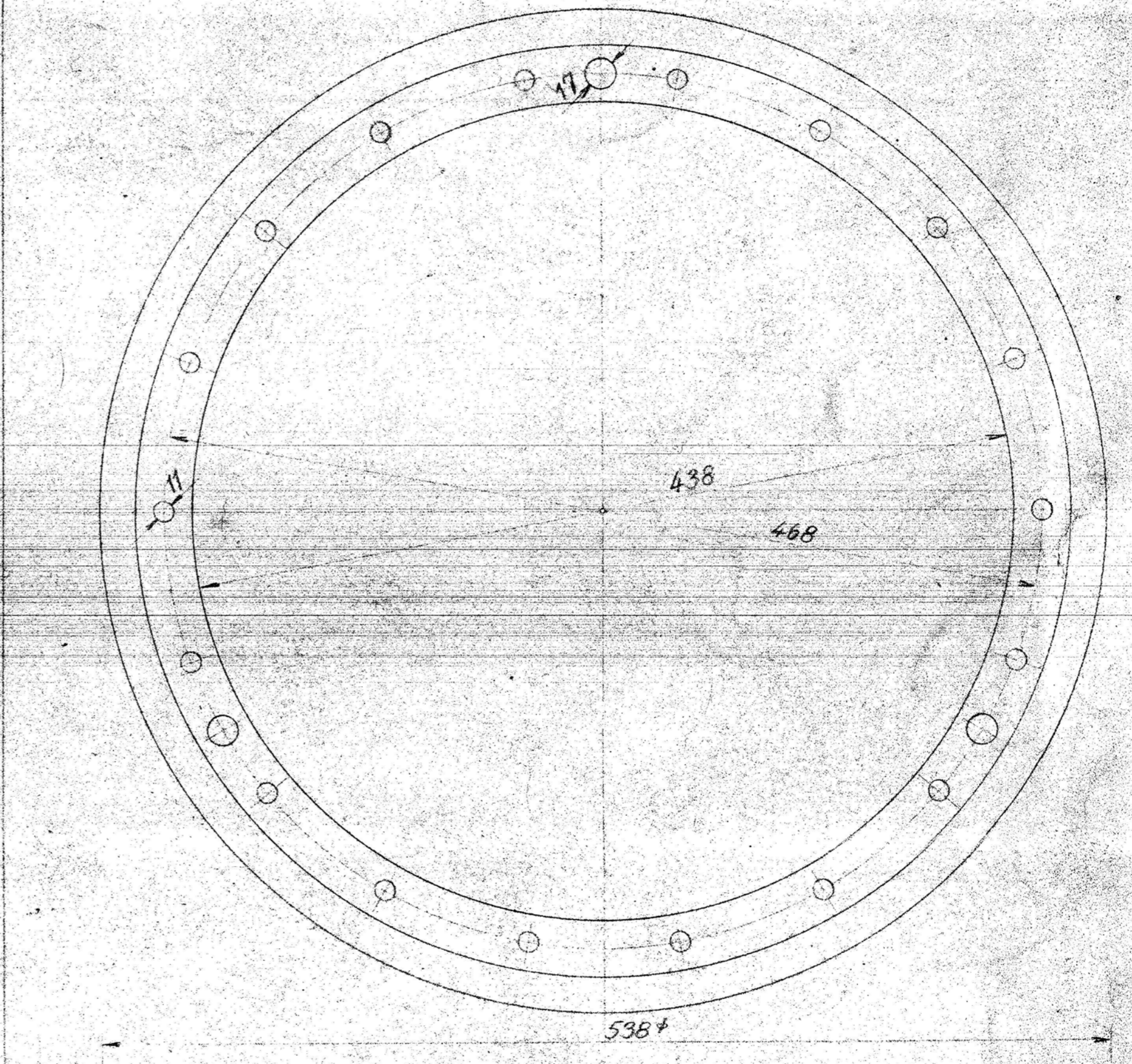
PR 7b Pos 14. Bundakse. 1Stk. 1:2 Rev. Flusjern.
