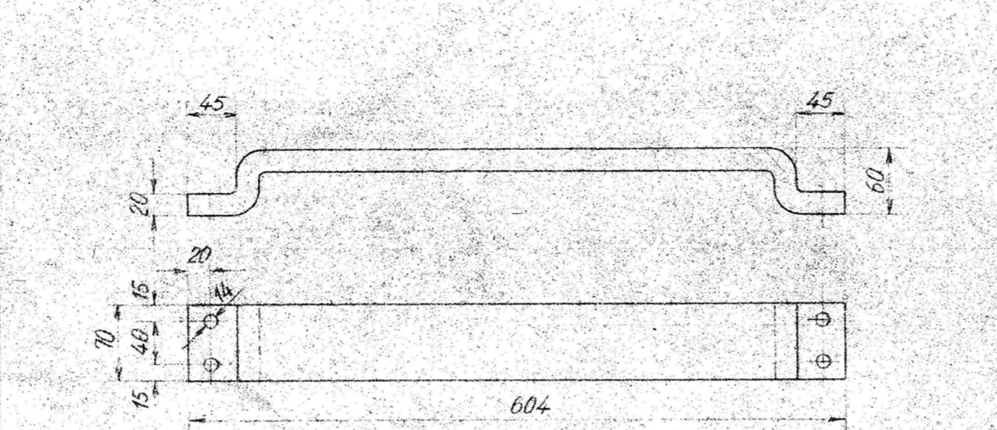
PR 7b Pos 11. Kontravægt. 2Stk. 1:5 Rev. Flusjern.
