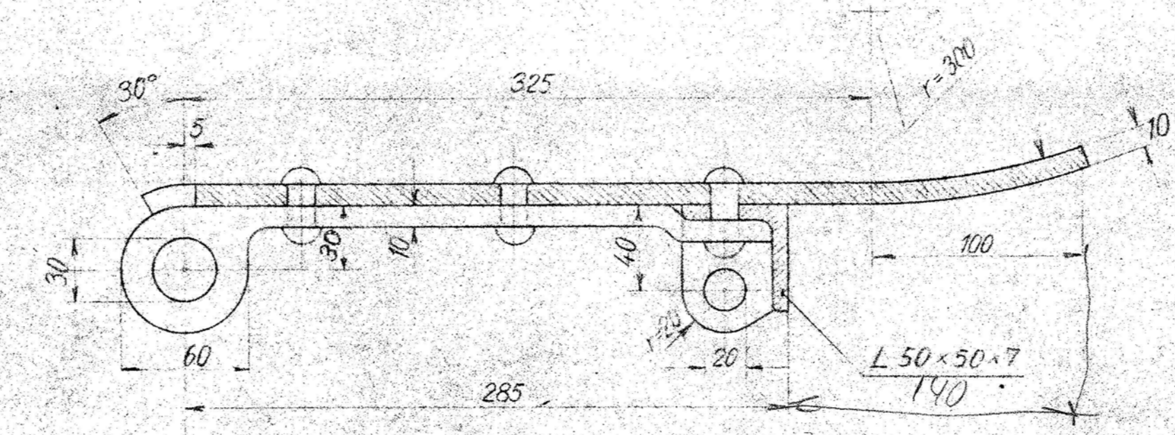
PR 7b Pos 2. Askefang. 1Stk. 1:25 Rev. Flusjern.
