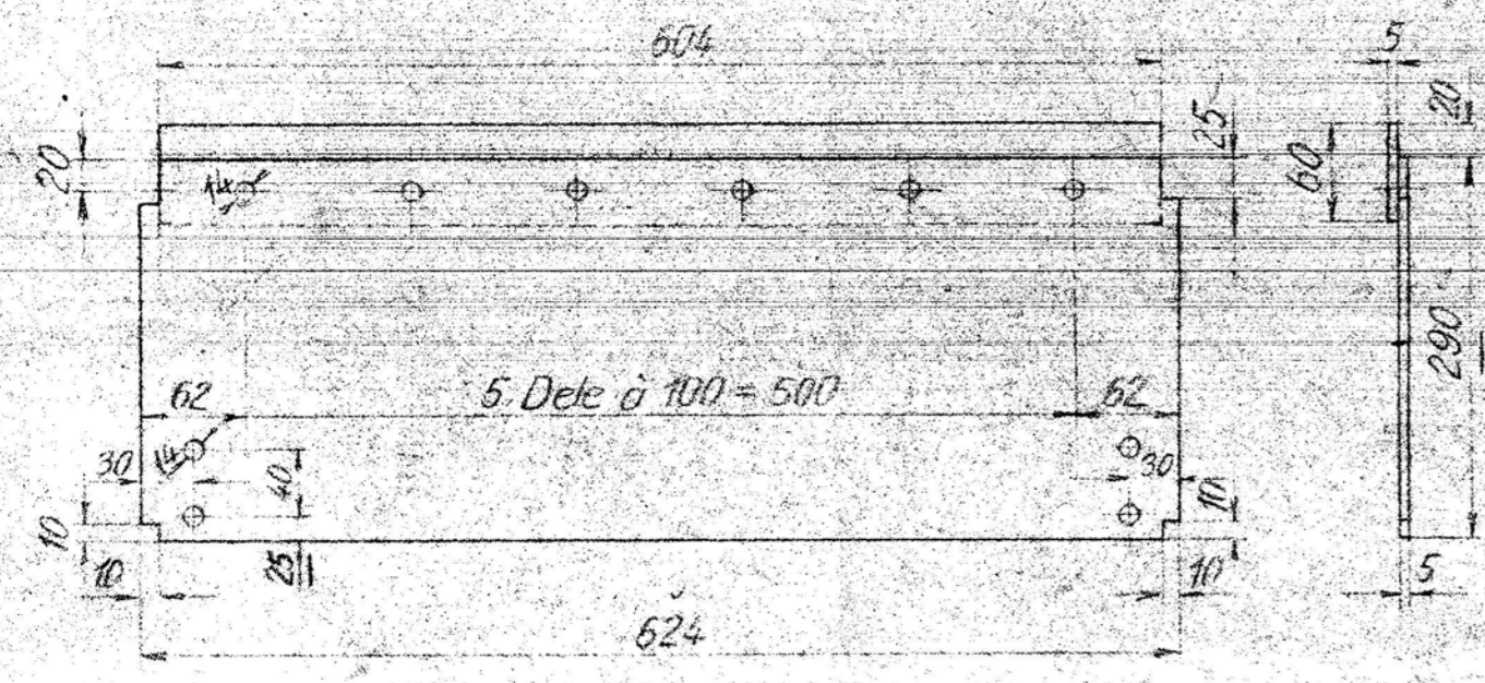
PR 7b Pos 6. Nederste Mel-klop. 1Stk. 1:5 Rev. Flusjern.
