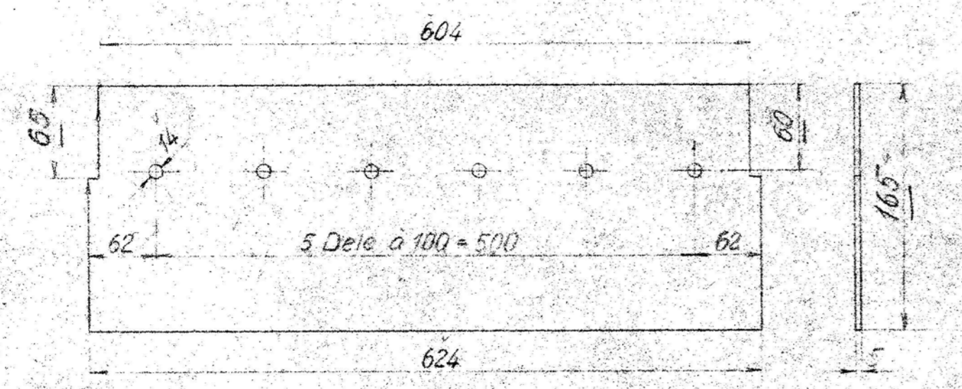
PR 7b Pos 5. Øverste Mel-klop. 1Stk. 1:5 Rev. Flusjern.
