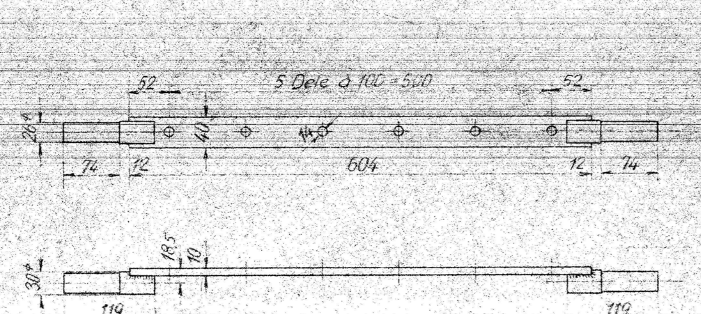
PR 7b Pos 10. Beslag. 2Stk. 1:5 Rev. Flusjern.
