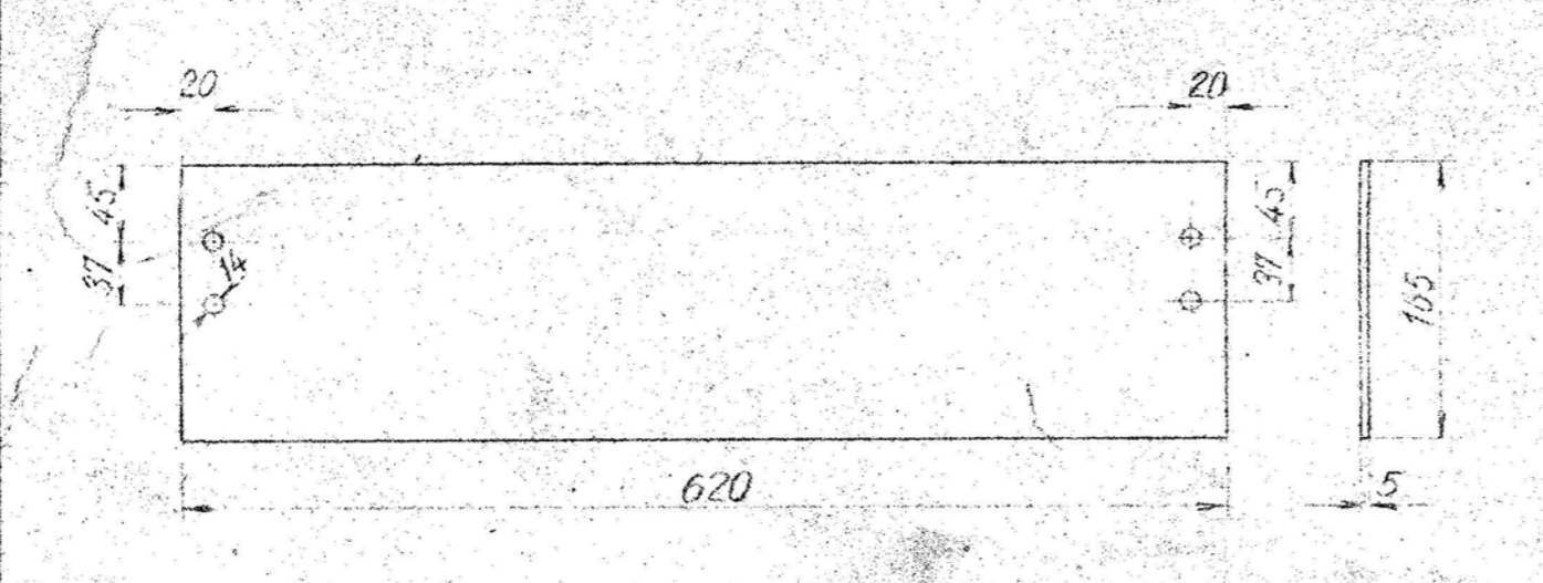
PR 7b Pos 12. Bagklap. 1Stk. 1:5 Rev. Flusjern.
