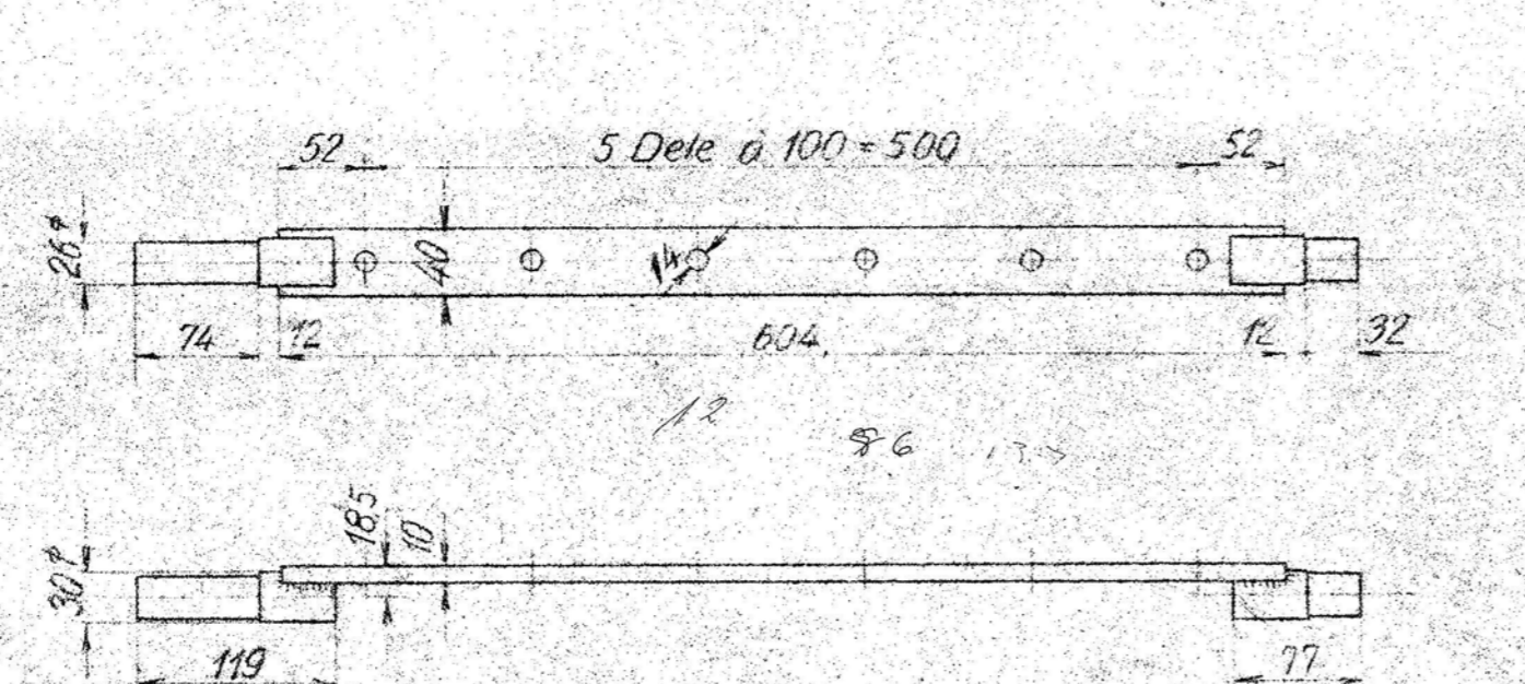
PR 7b Pos 9. Beslag. 2Stk. 1:5 Rev. Flusjern.
