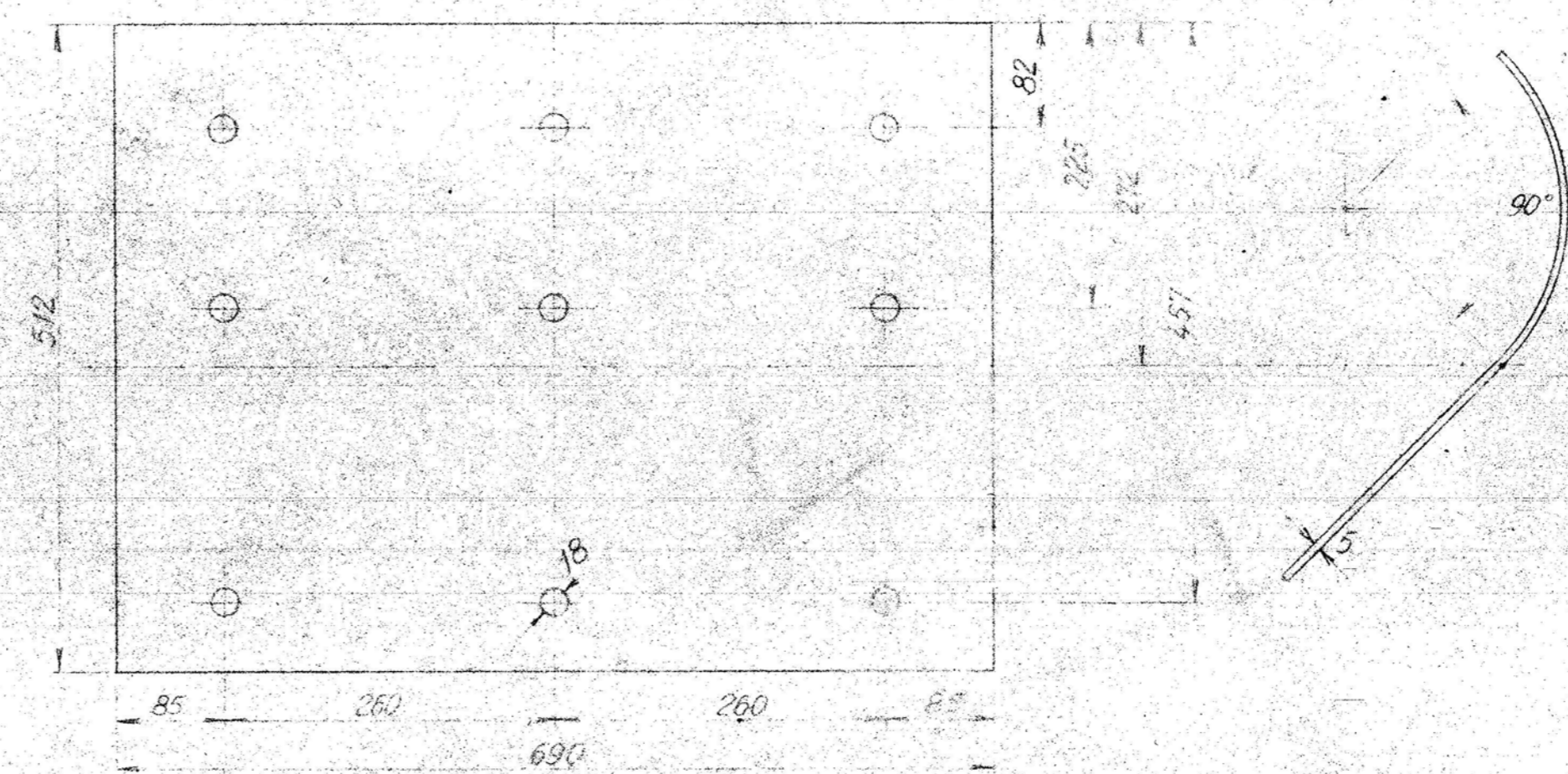
PR 7b Pos 3. Beskyttelsesplade 1Stk. 1:5 Rev. Flusjern.
