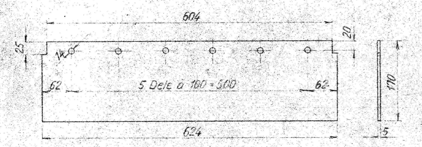
PR 7b Pos 7. Øverste Forklop. 1Stk. 1:5 Rev. Flusjern.
